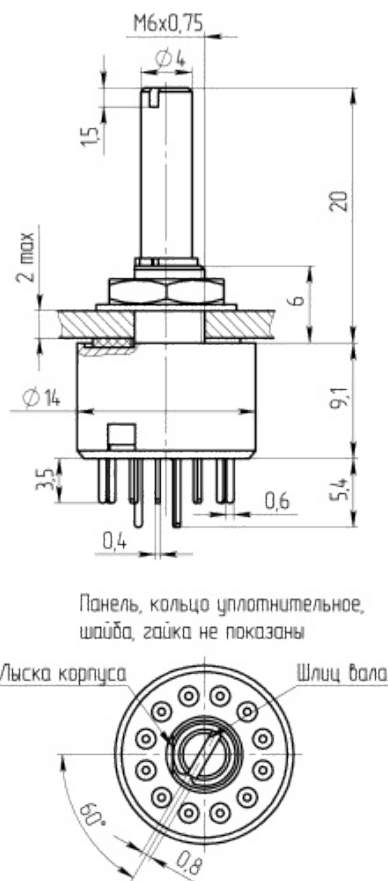
Габаритные и установочные размеры
