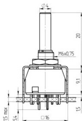
Габаритные и установочные размеры
