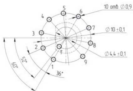
Разметка для крепления на плиту (вид со стороны вала)
