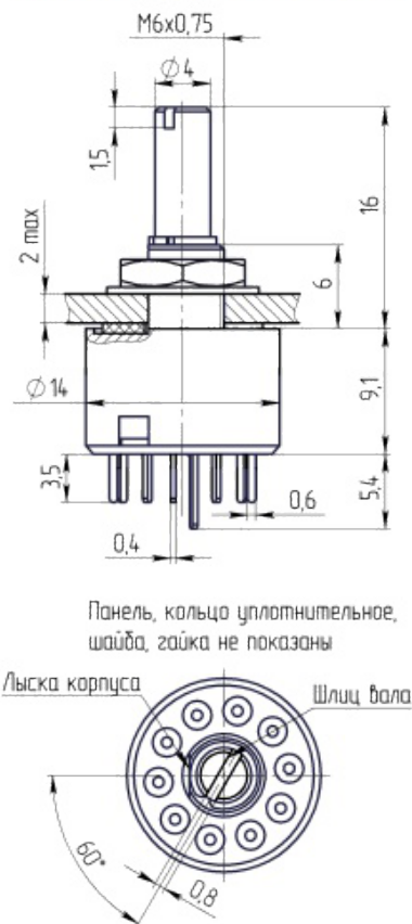
Габаритные и установочные размеры
