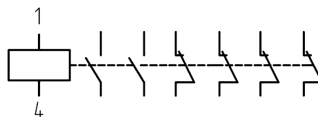
Электрическая принципиальная схема
