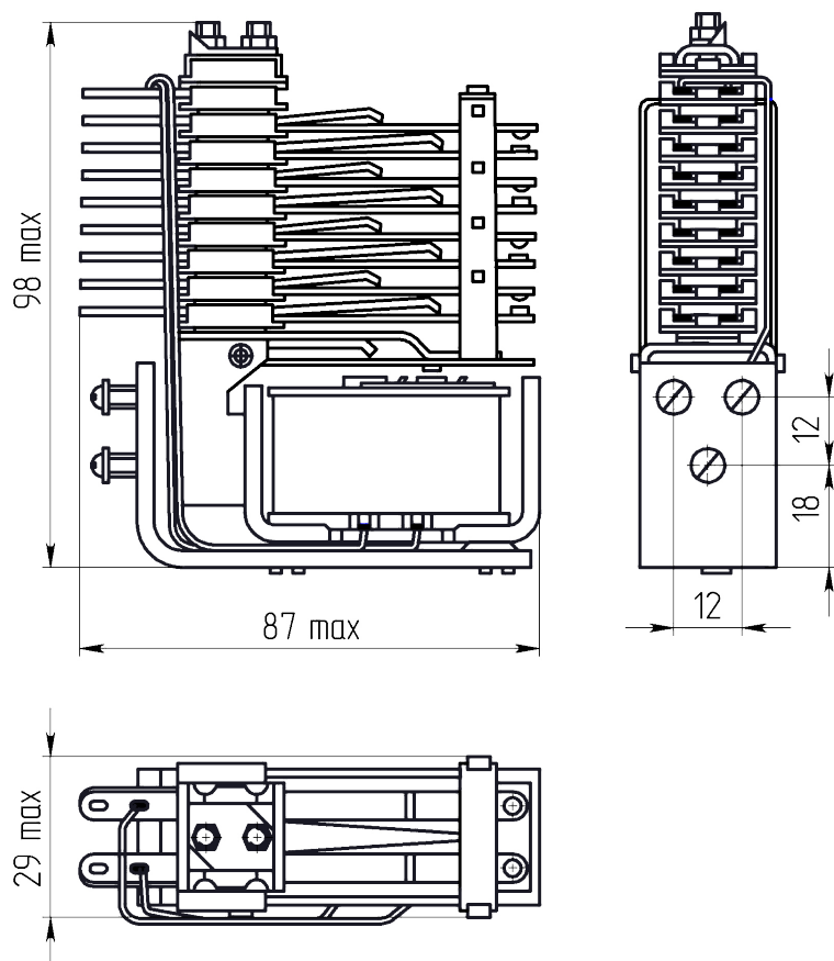
Габаритные и установочные размеры
