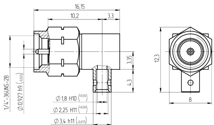
Габаритные и установочные размеры
