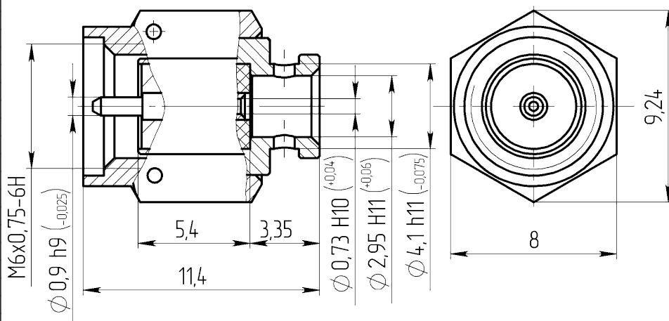
Габаритные и установочные размеры
