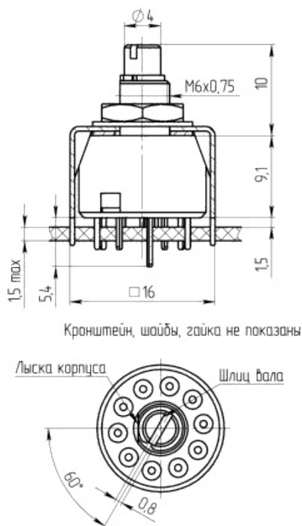
Габаритные и установочные размеры
