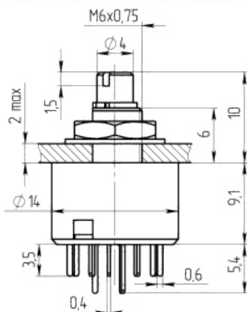
Габаритные и установочные размеры
