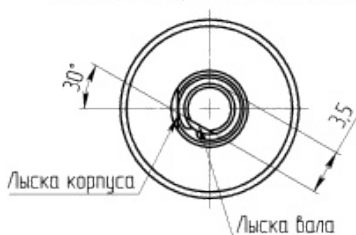
Панель, шайба, гайка не показаны
