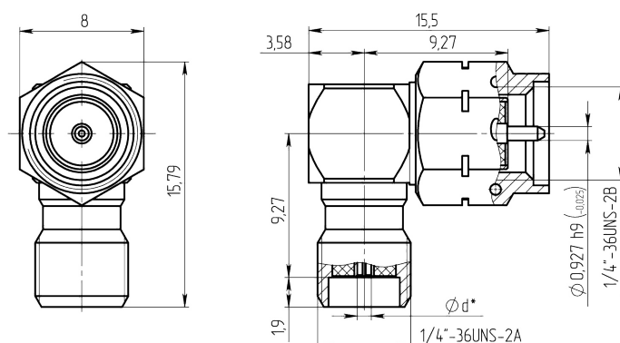
Габаритные и установочные размеры
