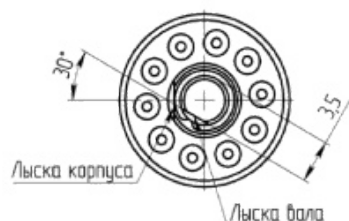
Панель, кольца уплотнительные, шайба, гайка не показаны
