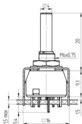
Габаритные и установочные размеры
