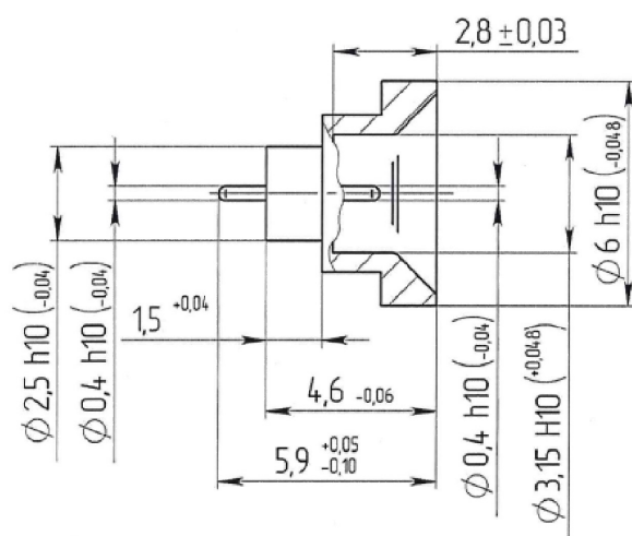
Габаритные и установочные размеры
