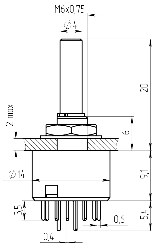
Габаритные и установочные размеры
