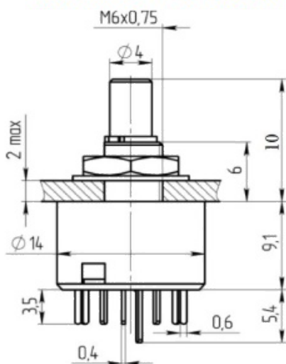
Габаритные и установочные размеры
