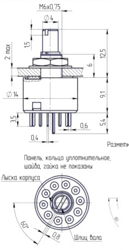
Габаритные и установочные размеры
