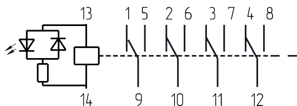
Электрическая принципиальная схема
