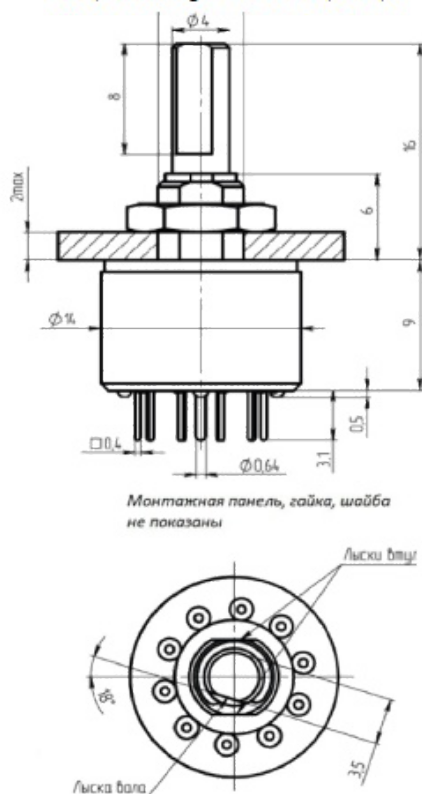
Габаритные и установочные размеры
